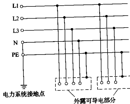
图 7 TN-S 系统
